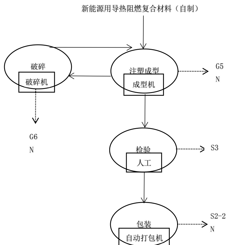
图2-4 5G通讯基站部件生产工艺流程图
