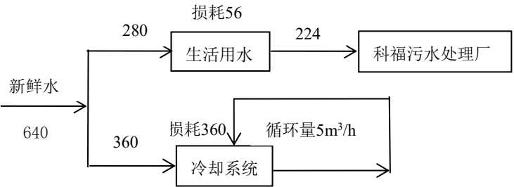
图2-1 全厂水量平衡图（单位：m 3 /a）
