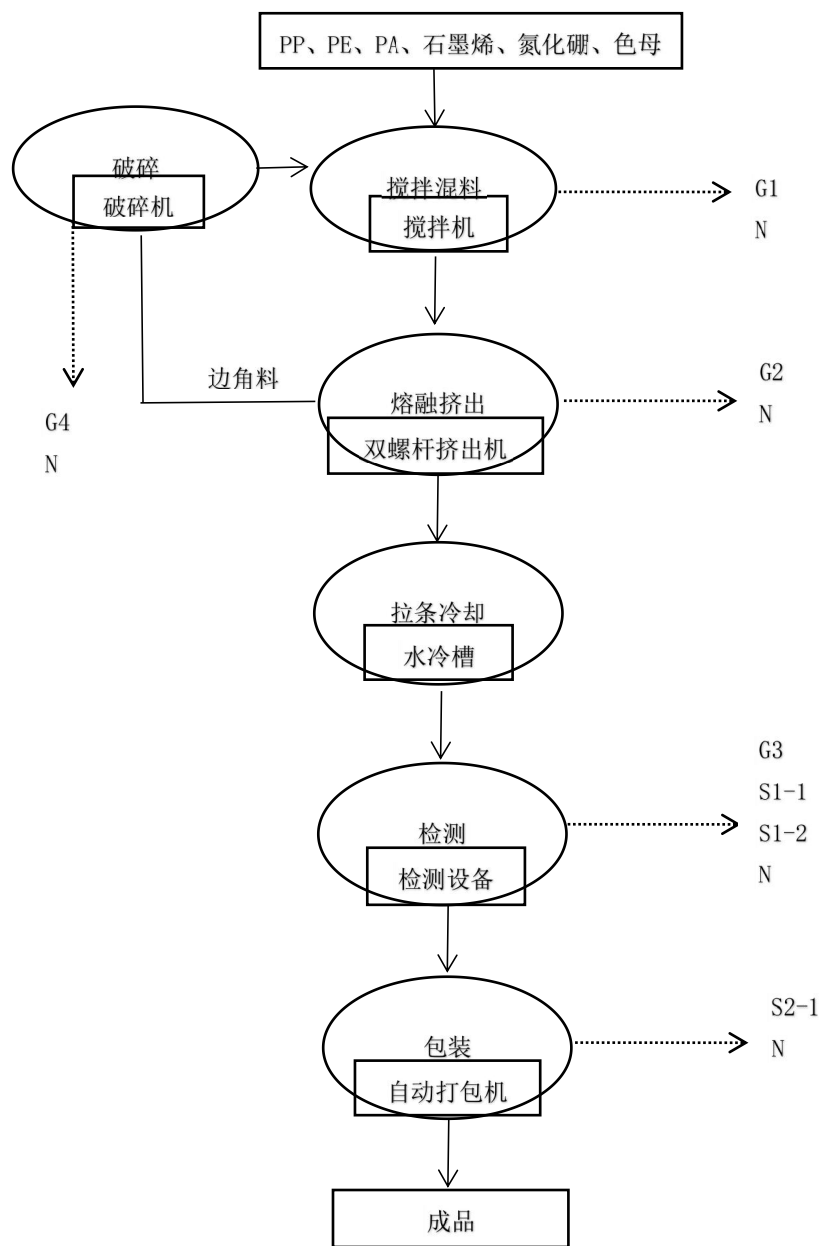
图2-3 新能用导热阻燃复合材料生产工艺流程图
