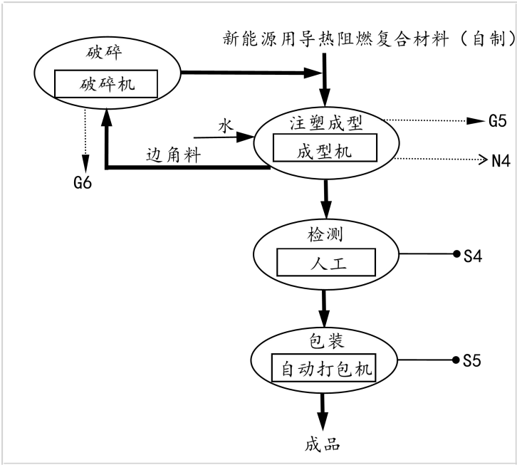
图2-6 5G通讯基站部件生产工艺流程图
