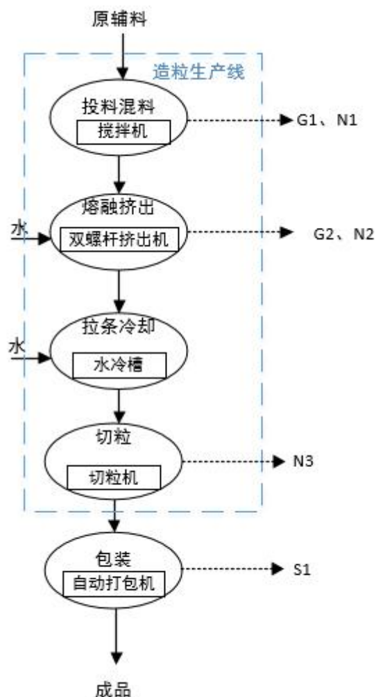
图2-5 新能源用导热阻燃复合材料生产工艺流程图
