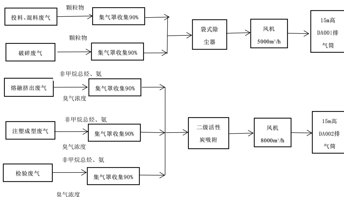
图4-1 废气收集处理系统示意图
